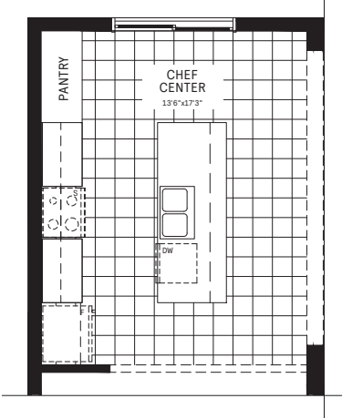
1 Chef Center
